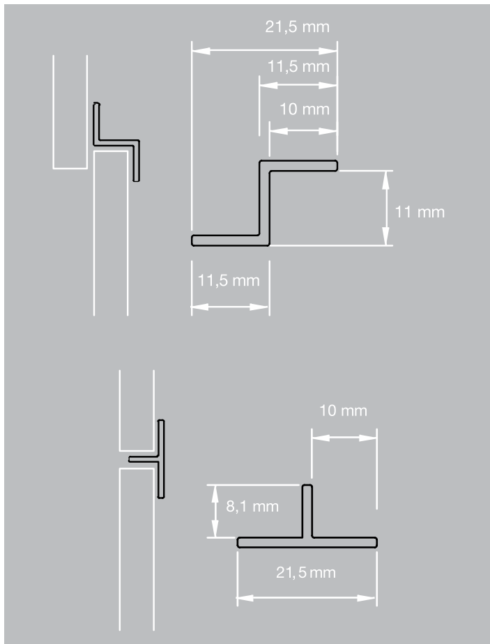
Perfil con forma Z y con forma T (Blanco / Cromo)
